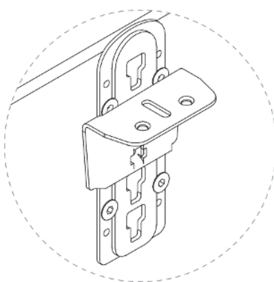
付属パーツを上向きに 取り付けた場合
