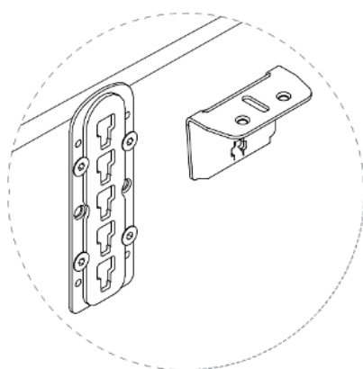
取り付け位置は 4段階
