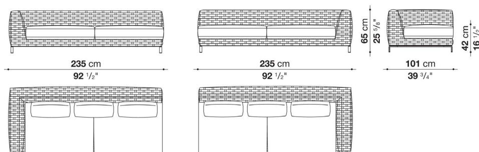
RF235S
