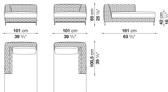
RF161LS
